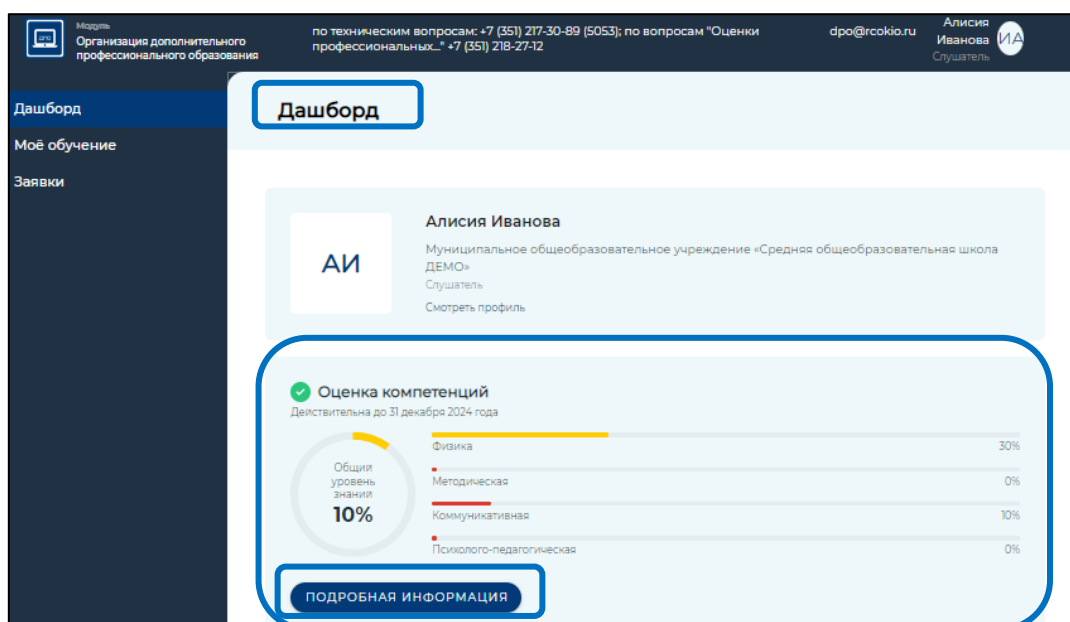
Рисунок 22. Раздел «Дашборд»
