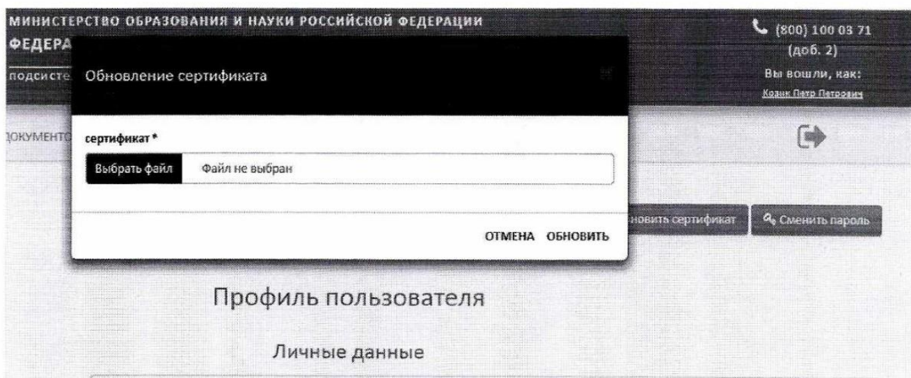
Рис. 5 – Обновление сертификата
