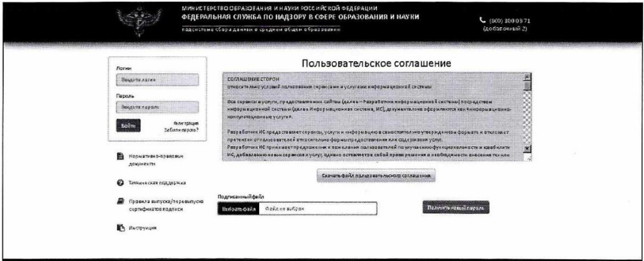
Рис. 3 – Восстановление пароля
